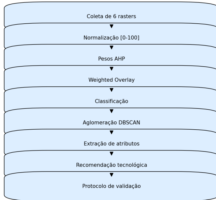
Figura 2: Fluxograma completo do processo de identificação: (A) Coleta de 6 rasters; (B) Normalização min-max [0-100]; (C) Aplicação de pesos AHP; (D) Weighted Overlay; (E) Classificação; (F) Aglomeração DBSCAN; (G) Extração de atributos; (H) Recomendação tecnológica por zona; (I) Protocolo de validação.
